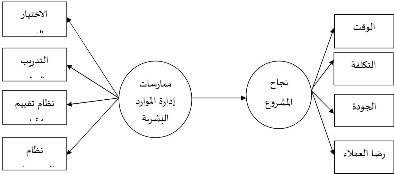
شكل 1: نموذج الدراسة
